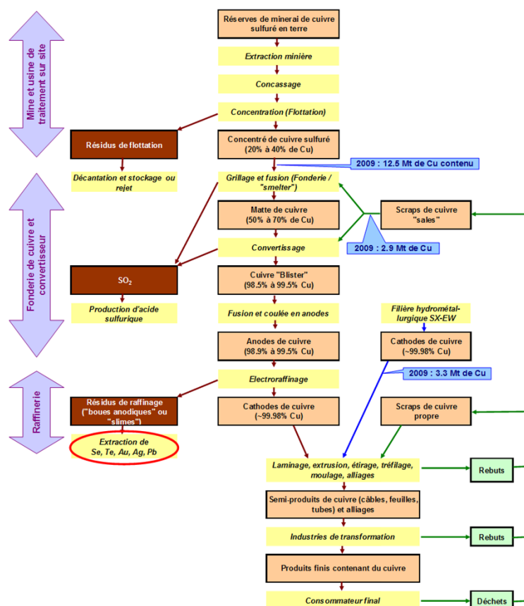
Schéma du processus de production du cuivre par pyroméallurgie
