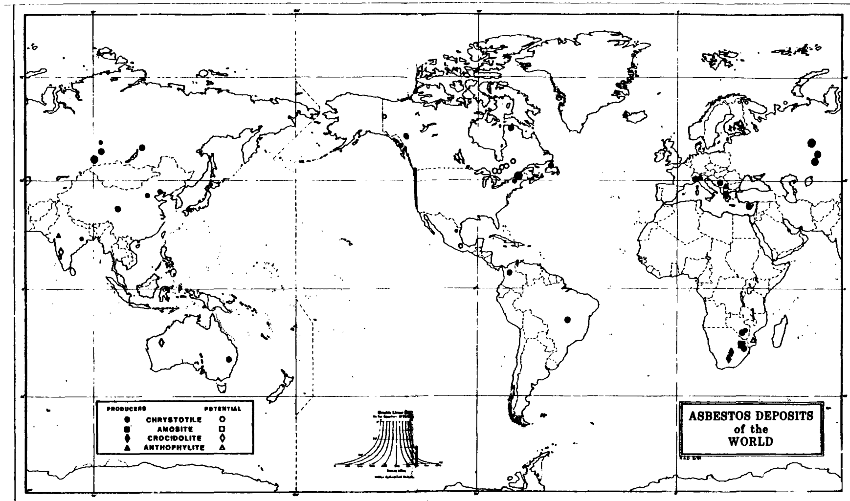
Figure 2 - Principaux gisements d'amiante dans le Monde.
